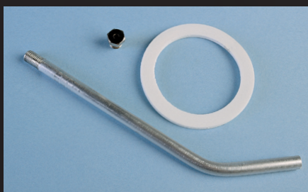
57310215 - Tubo de absorción 57212214 - Prensa-estopas de producto 50810229 - Junta de cierre del depósito
